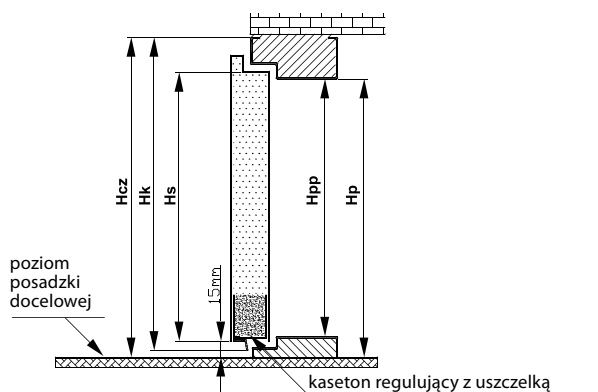
Wymiary przy całkowicie ukrytym kasetonie regulacyjnym
