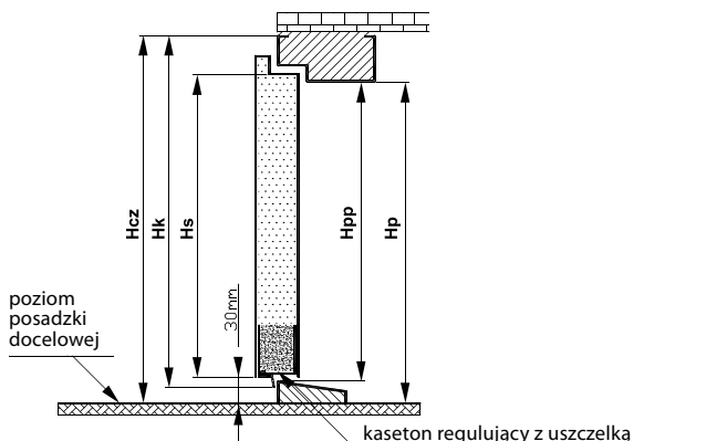
Wymiary przy całkowicie ukrytym kasetonie regulacyjnym
