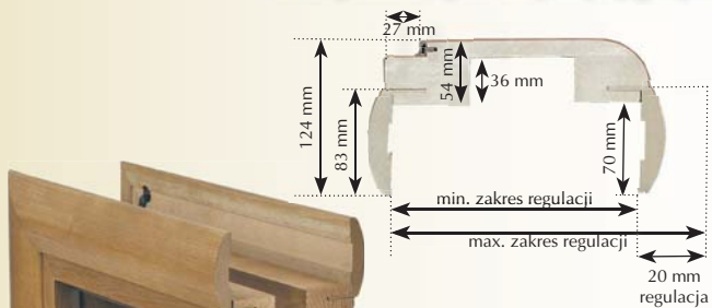
Przekrój ościeżnicy do skrzydeł przylgowych
