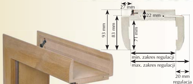
Przekrój ościeżnicy do skrzydeł bezprzylgowych
