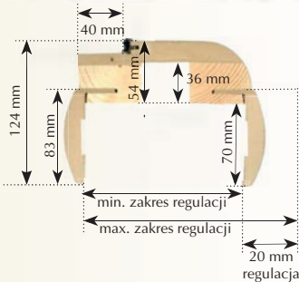
Przekrój ościeżnicy do skrzydeł bezprzylgowych
